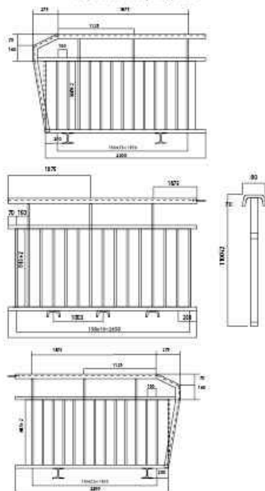
Перильное ограждение
